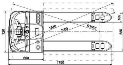
CBD20-150
