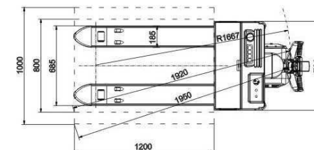
CBD20-100
