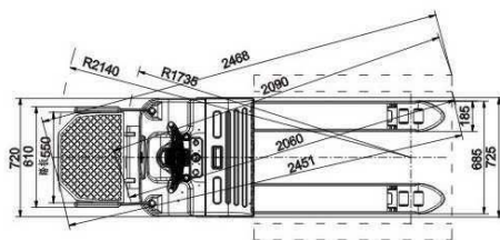
CBD20-470
