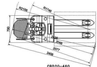
CBD20-460
